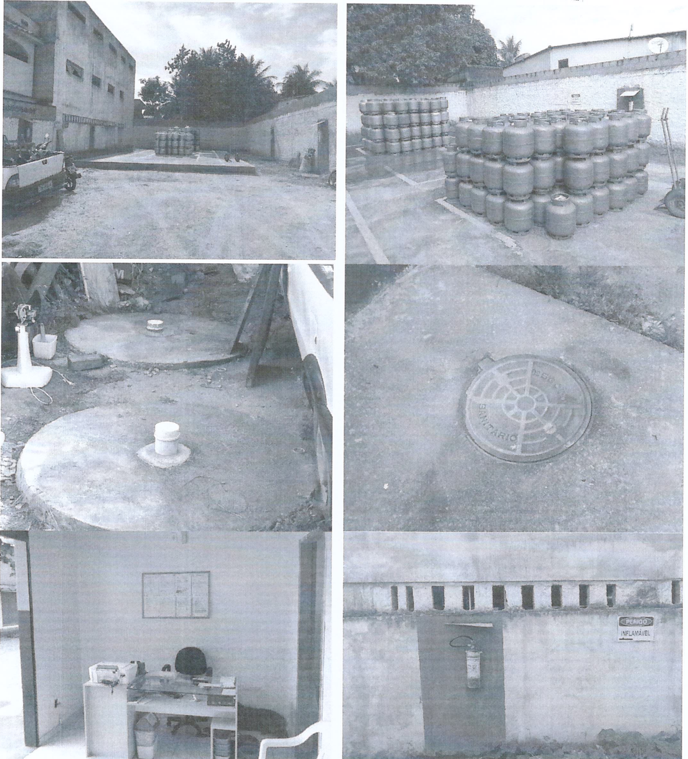
Figura 3: (A) e (B) Pátio de estocagem de botijões. (C) e (D) Sistema de esgotamento sanitário. (E) Escritório e (F) Extintor de incêndio.
