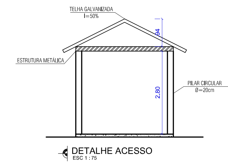
DETALHE ACESSO ESC 1:75
