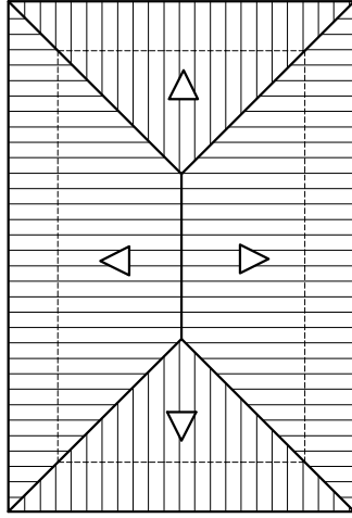
COBERTURA - CONST. I ESCALA 1/75
