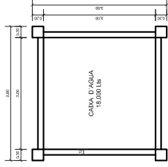
PLANTA BAIXA 2 - CX D'AGUA ESCALA 1/50
