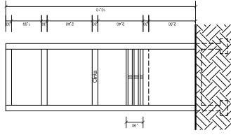
FACHADA - CX D'AGUA ESCALA 1/75
