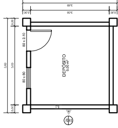
PLANTA BAIXA 1 - CX D'AGUA ESCALA 1/50
