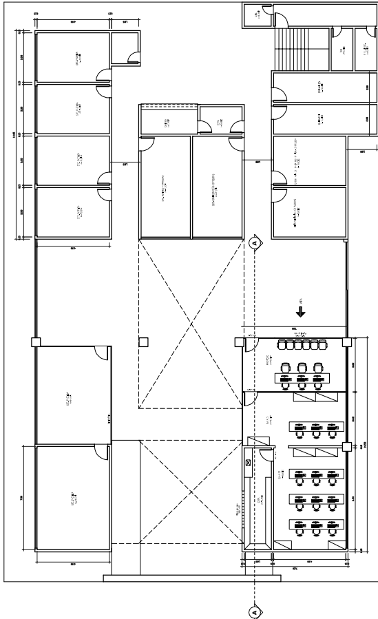
Planta Baixa - Situação Final Esc. 1:200
