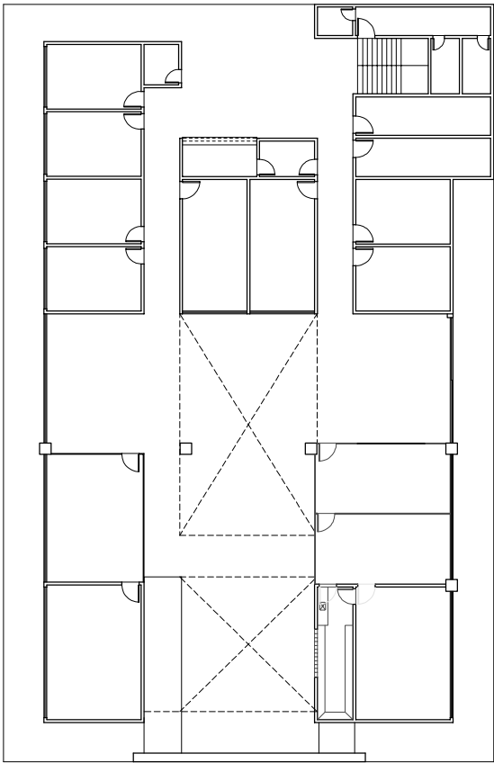
Planta Baixa - Reforma Esc. 1:200
