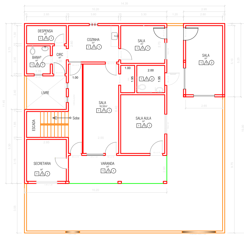
Pavimento Térreo ESC 1:125
